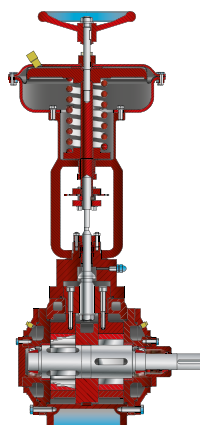
ACTUATOR
